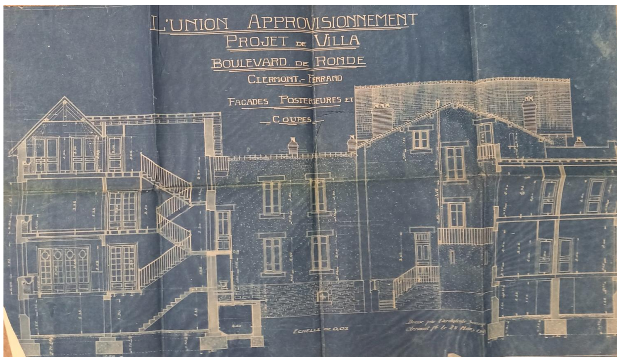
Coupe transversale et élévation postérieure
