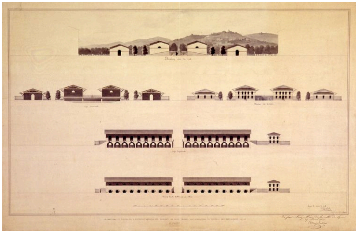
Elévation et coupe, premier projet de l'entrepôt des liquides
