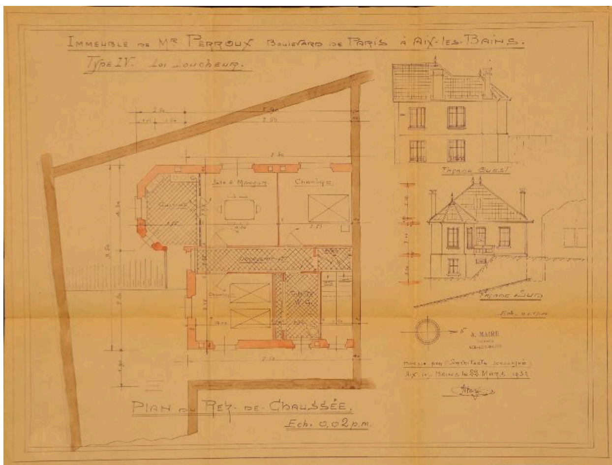
Plan du Rez-de-chaussée. Façade ouest. Façade sud
