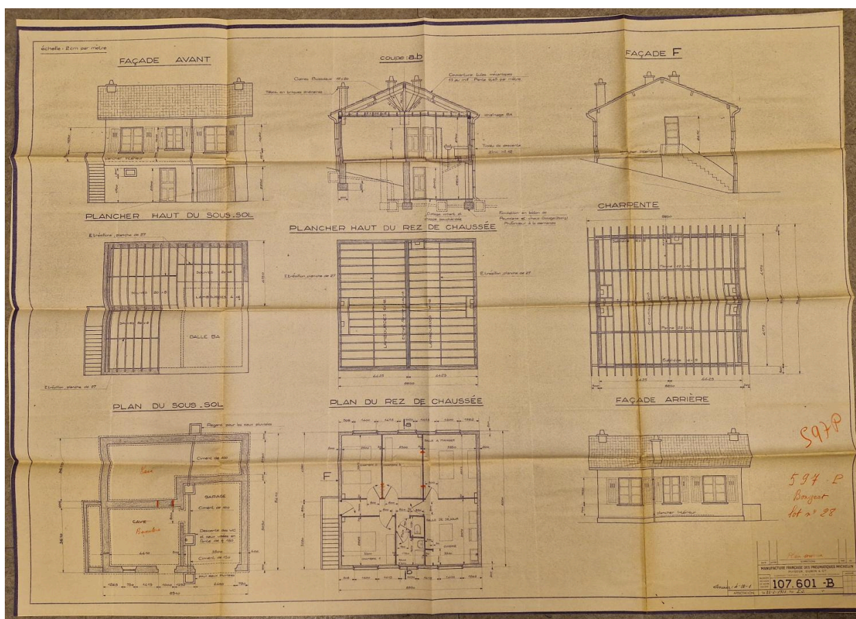
Plans, coupe, élévations d'une habitation "Castor" semi-enterrée à deux niveaux, allée des Castors, 1953.
