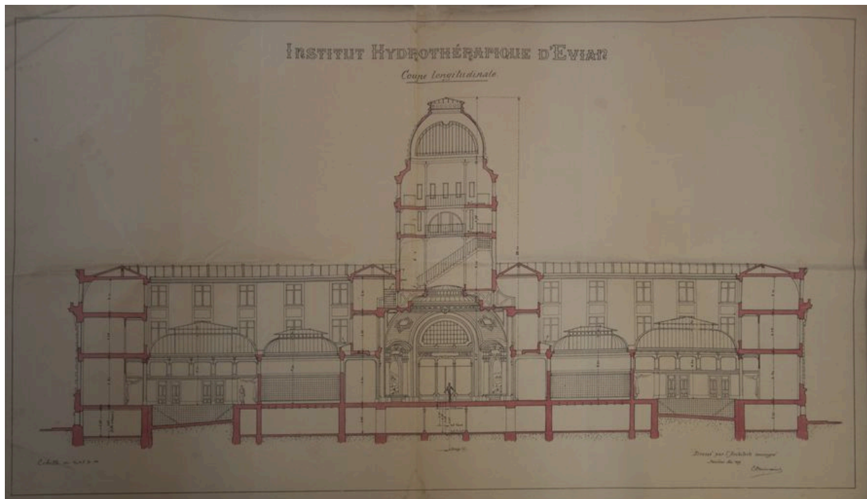
Institut Hydrothérapique d'Evian. Coupe longitudinale, novembre 1899. Plan. Archives départementales de la Haute-Savoie © Archives départementales de la Haute-Savoie. 2 O 946
