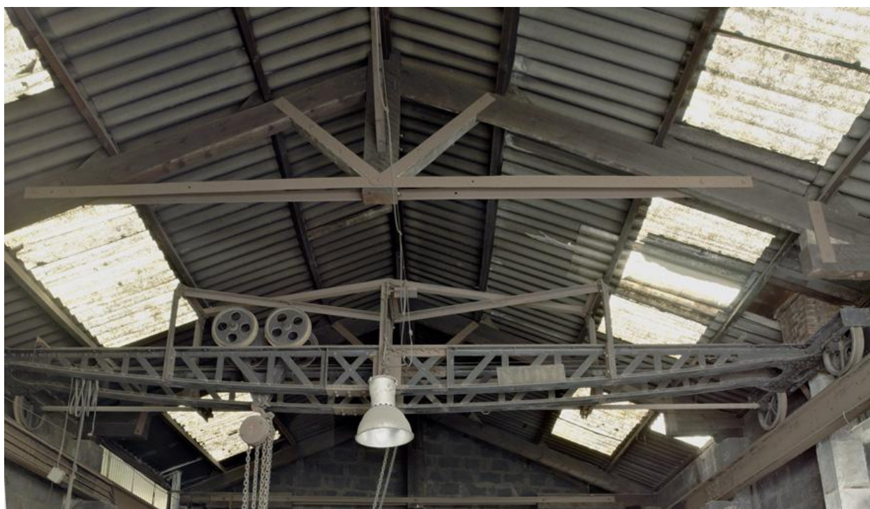
Charpente métallique des ateliers
