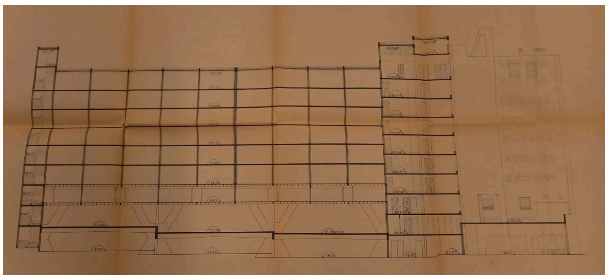
Coupe longitudinale
