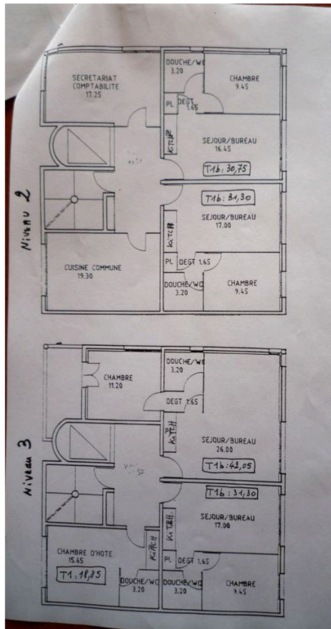
Maison paroissiale : plan du deuxième et du troisième étage
