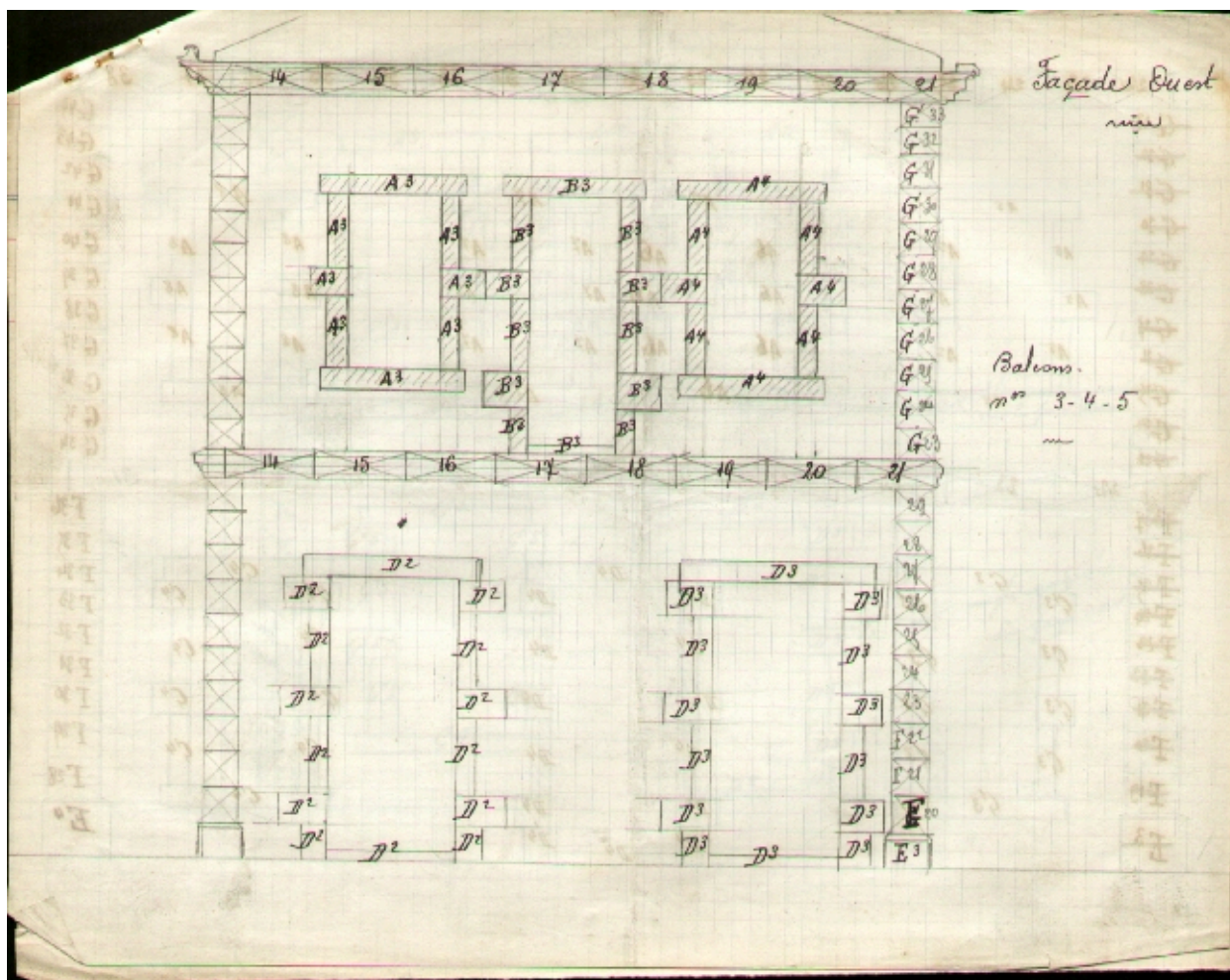
Elévation ouest
