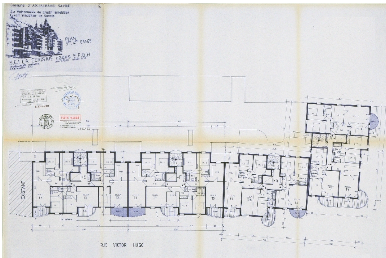
Plan des 3e et 4e étages, cages E, F, G et H
