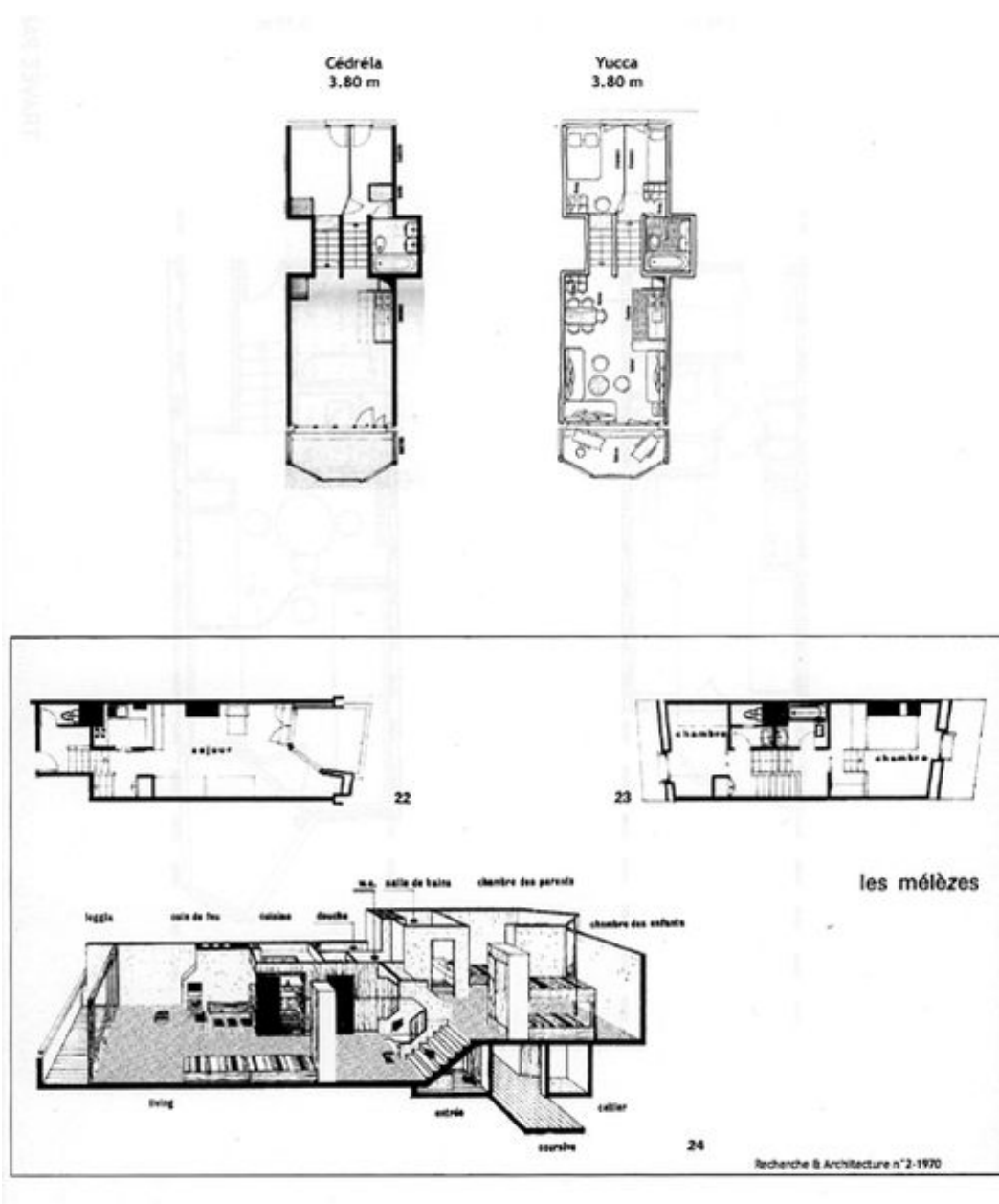
Plan d'un appartement d'une travée. Relevé schématique
