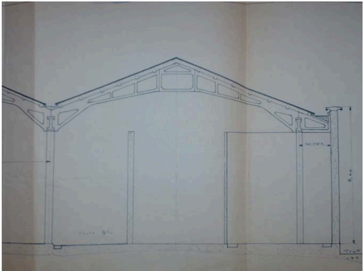
Plan de l'Ecole Française de Tannerie ; Locaux d'enseignement ; plan de coupe 3
