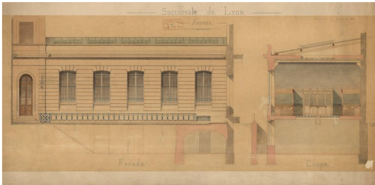
Elévation et coupe de l'annexe construite dans la cour (1892) (Banque de France, service du Patrimoine Historique et Artistique, non coté, dessin de Jean-Claude Merlin).
