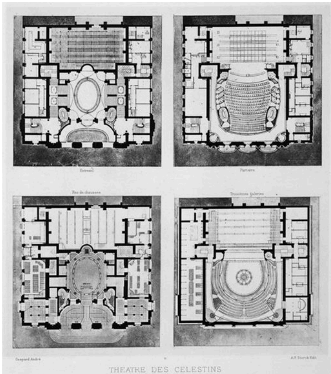
Théâtre de Gaspard André : plans, estampe dans L'Oeuvre de Gaspard André, Lyon : A. Storck, 1898, pl. 11
