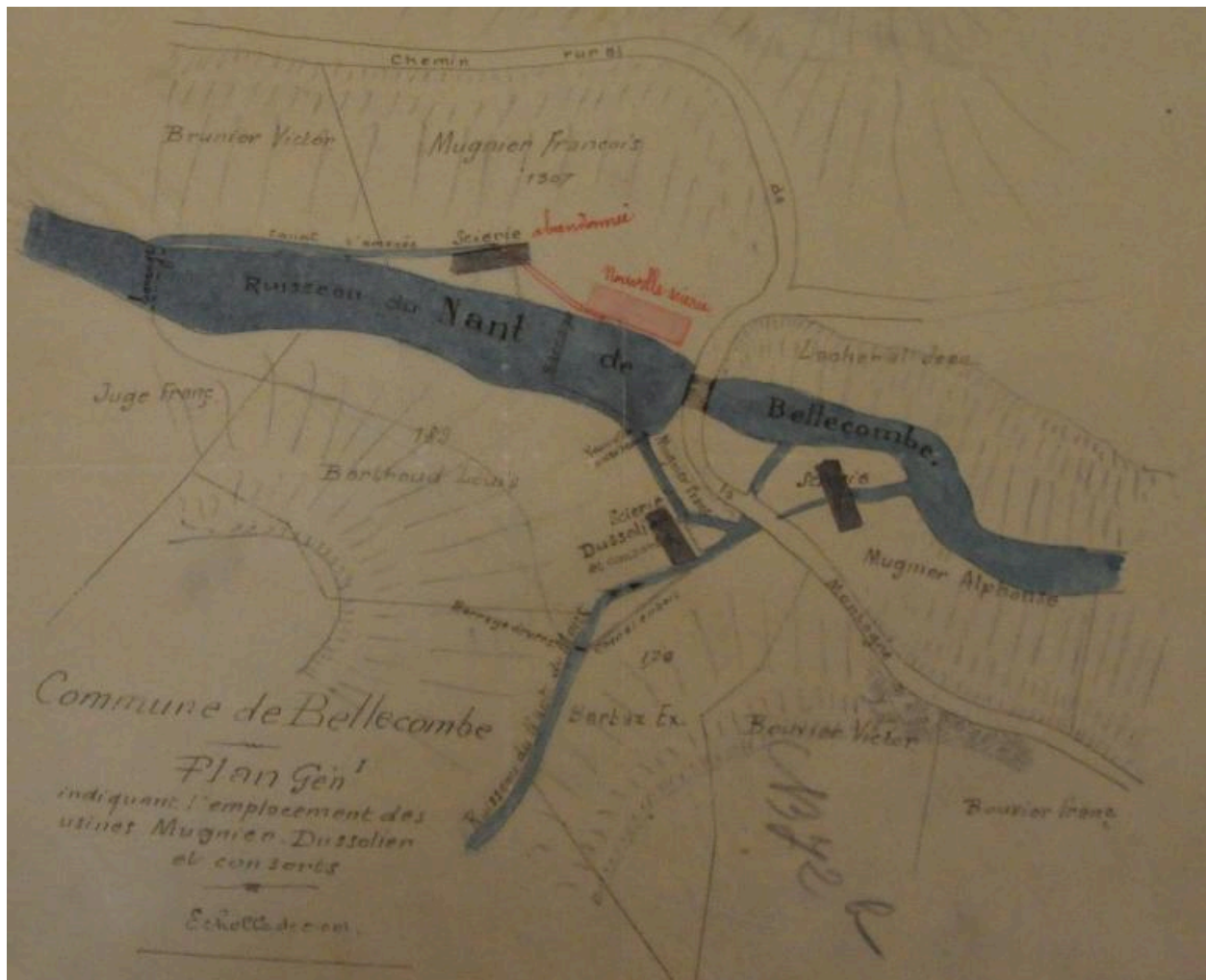
Plan accompagnant la demande de déplacement de la scierie, 1895 (FR.AD073, 45SPC2).
