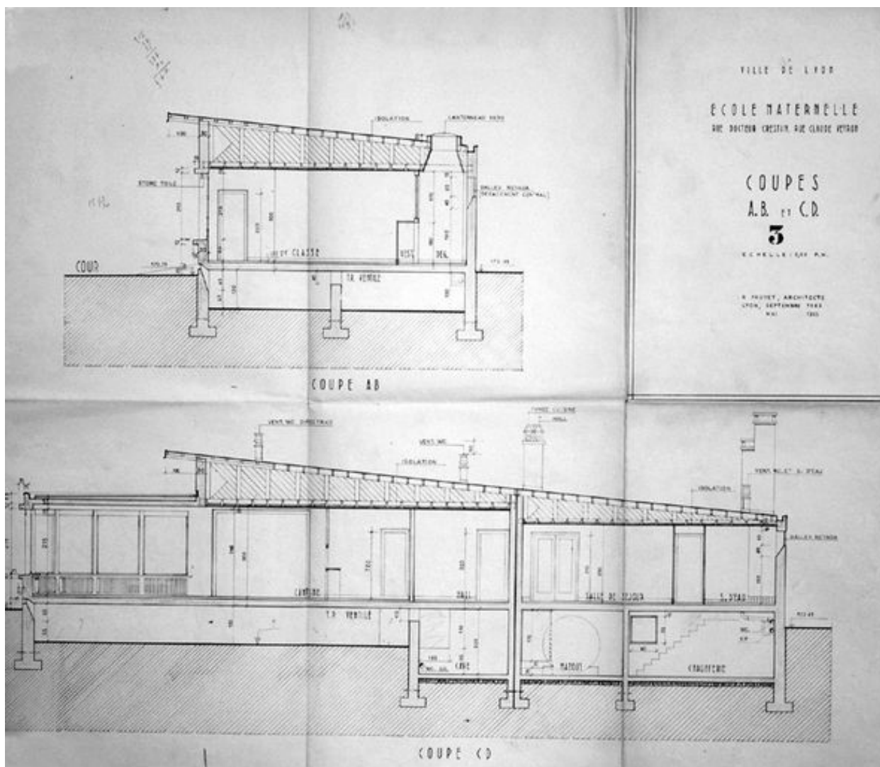
Coupes AB et CD, R. Fauvet architecte. 1:50, mai 1965
