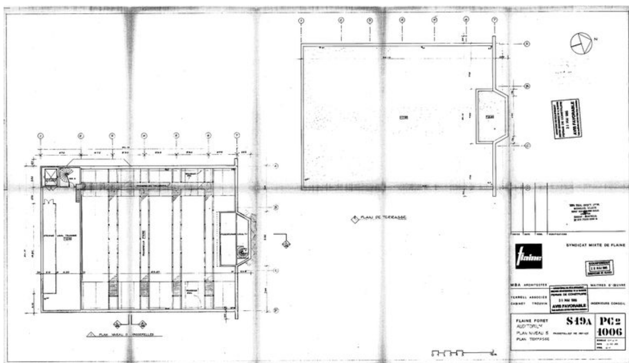
Plan du niveau 5, passerelle de service. Plan de la terrasse. MBA architectes, Terrell associés, 10 mai 1985 (AC Arâches-la-Frasse)
