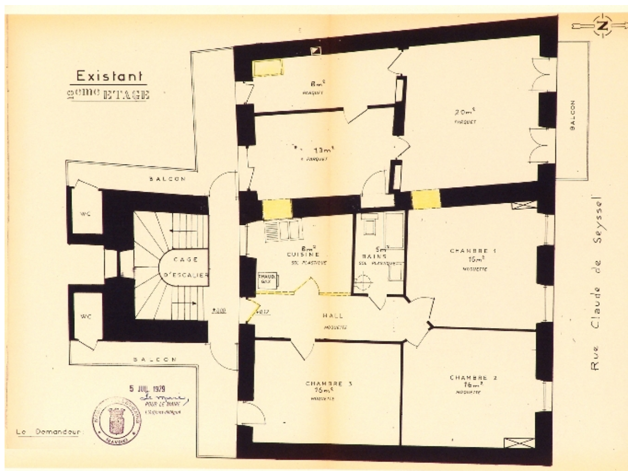
Plan du 2e étage avant travaux
