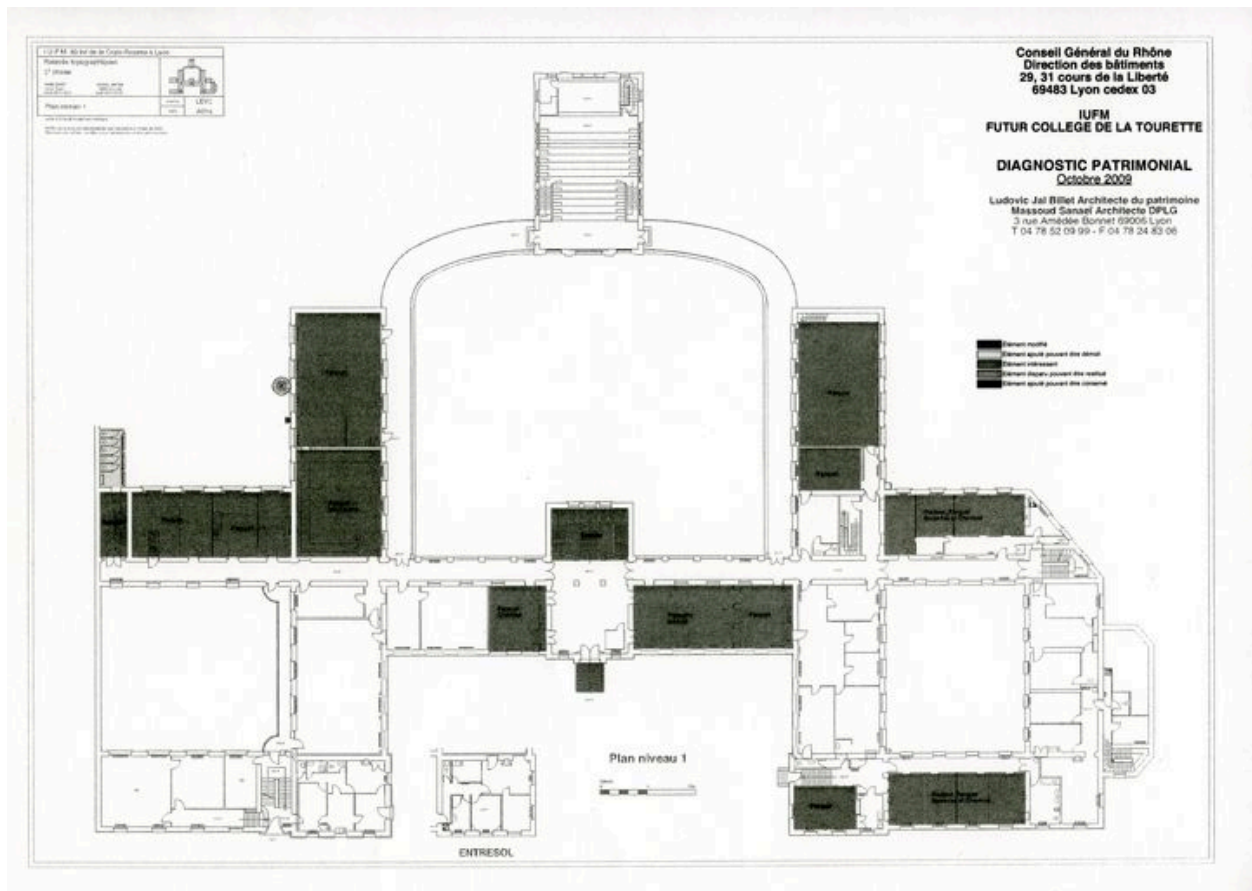
Plan du rez-de-chaussée, dit étage des classes (2009) (Conseil général du Rhône, Ludovic Jal-Billet, tirage d'architecte).
