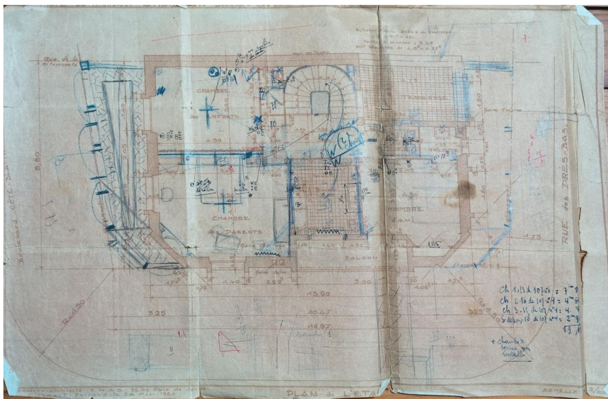
Plan de l'étage (plans modificatifs 1934)
