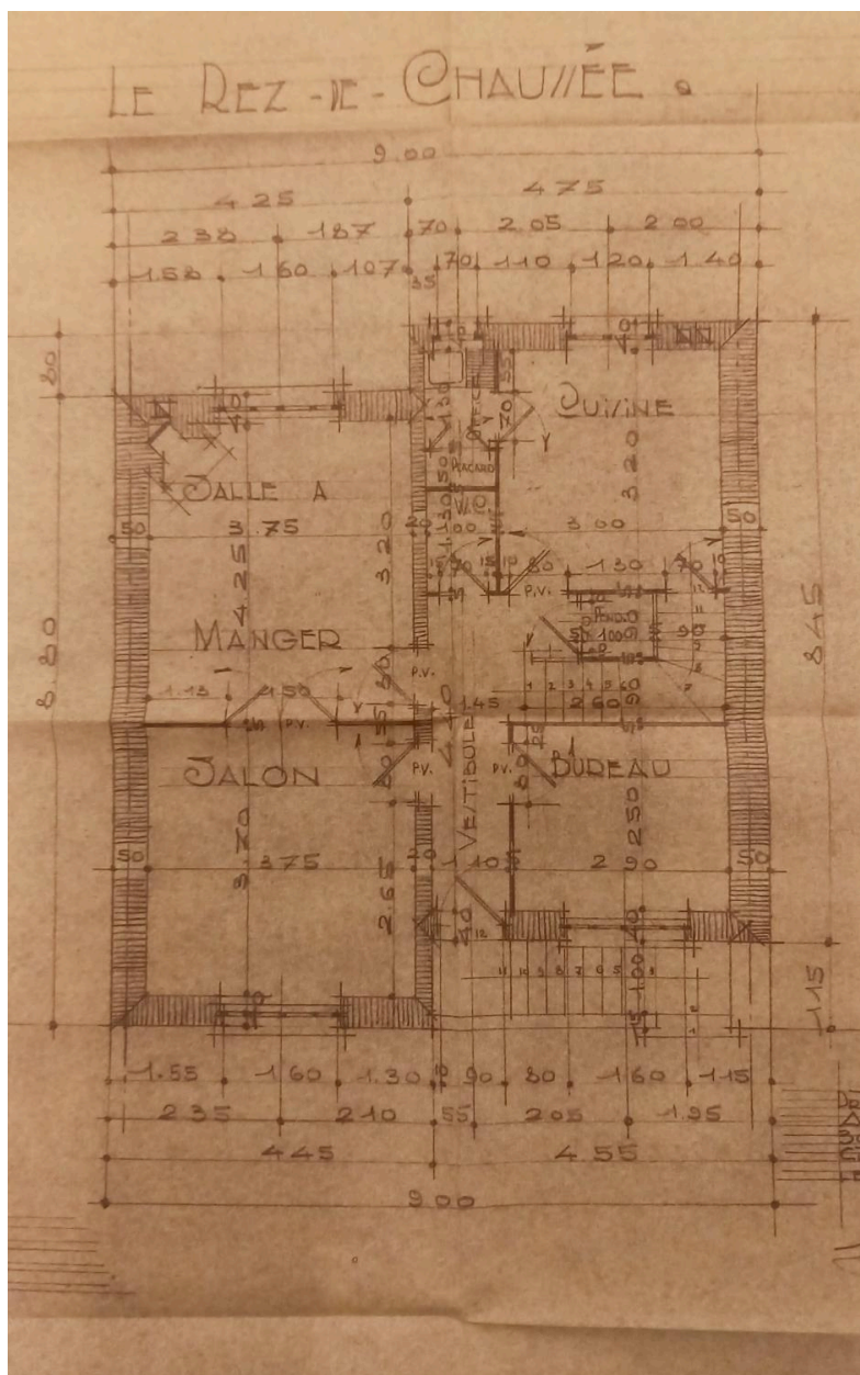
Plan du rez-de-chaussée
