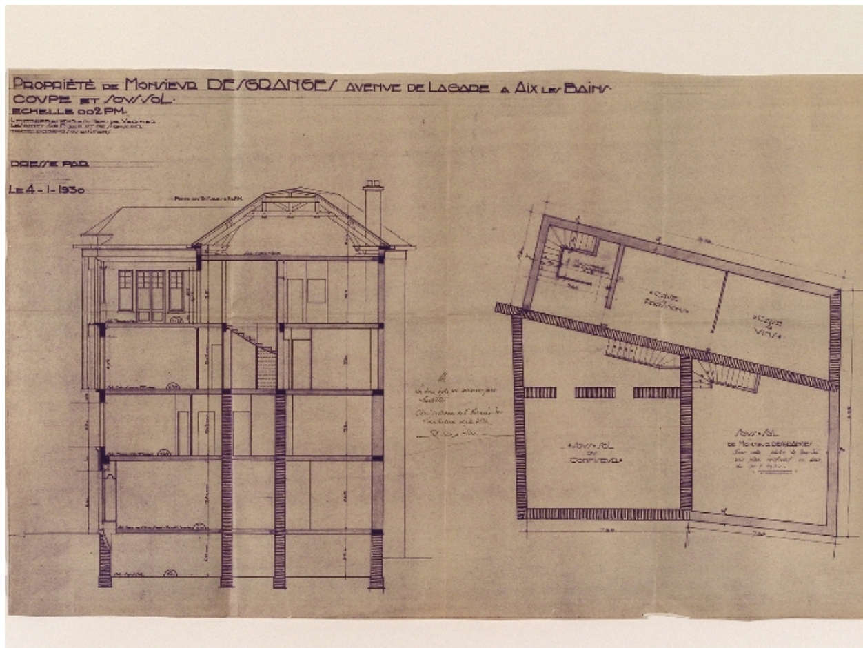
Plan du sous-sol et coupe
