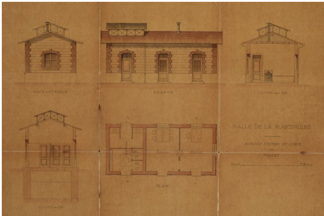
Halle de la Martinière, bureau d'octroi et lieux d'aisance, projet
