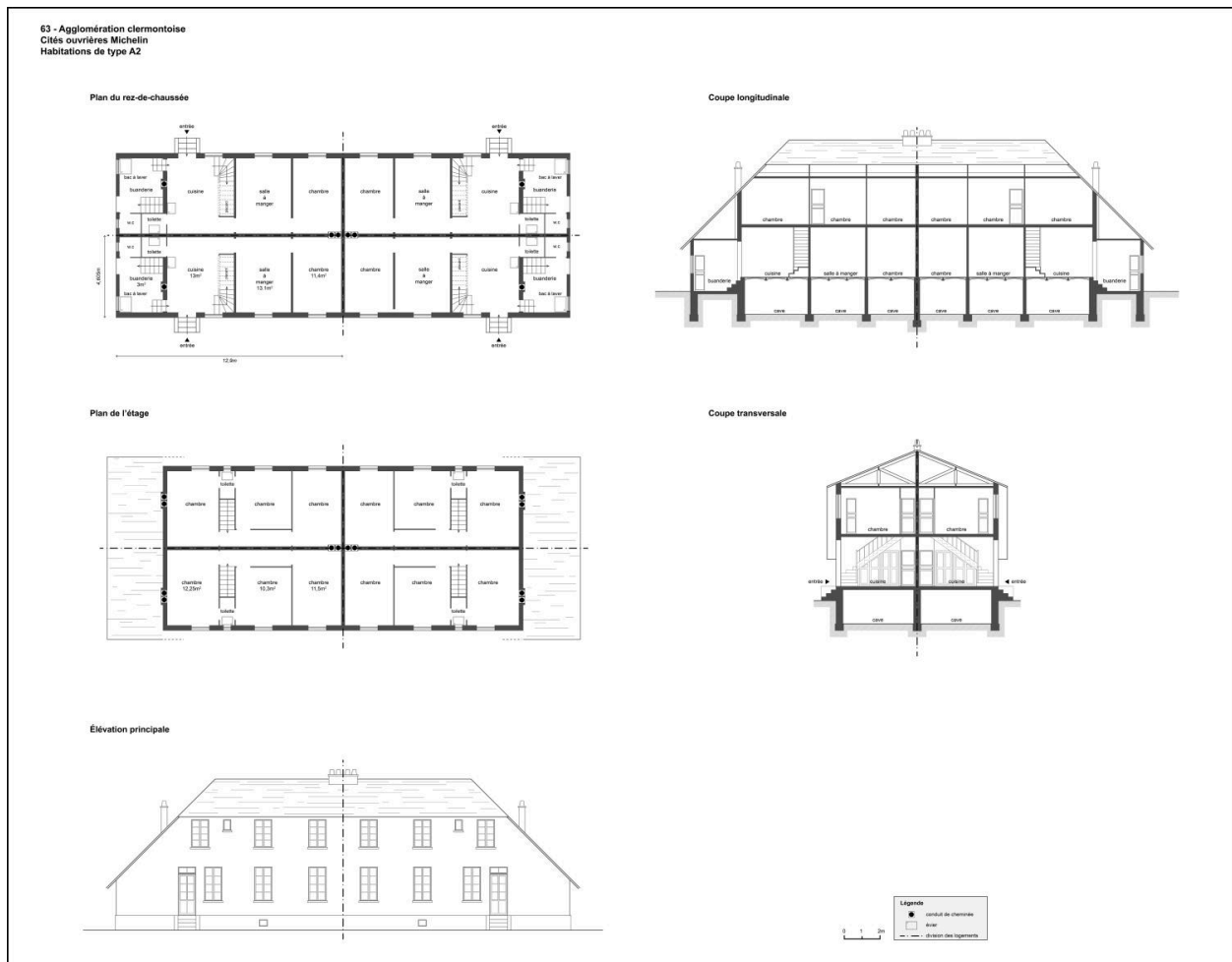
Plan des habitations de type A2.
