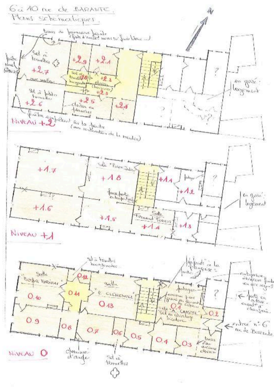
Plans schématiques des étages 0 à +2 et annotations de terrain.
