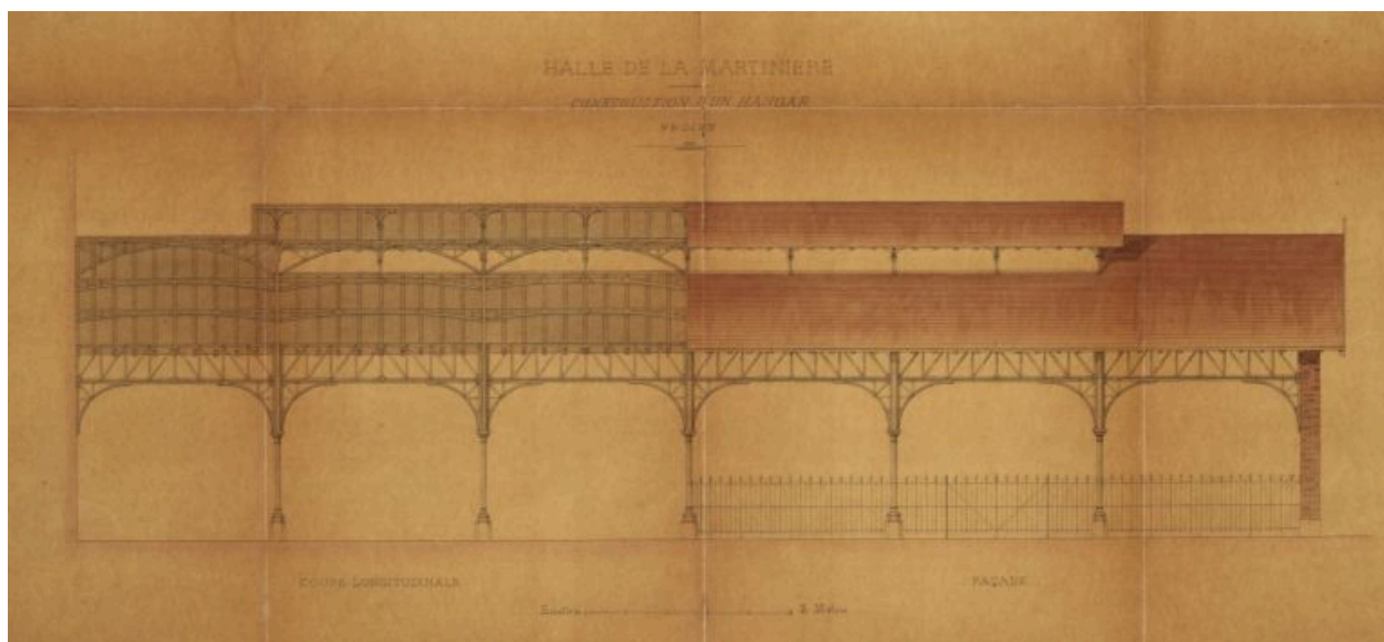
Halle de la Martinière, construction d'un hangar, projet, coupe longitudinale
