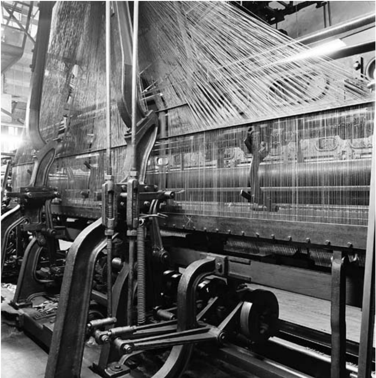
Vue arrière passage fils métier Johnson
