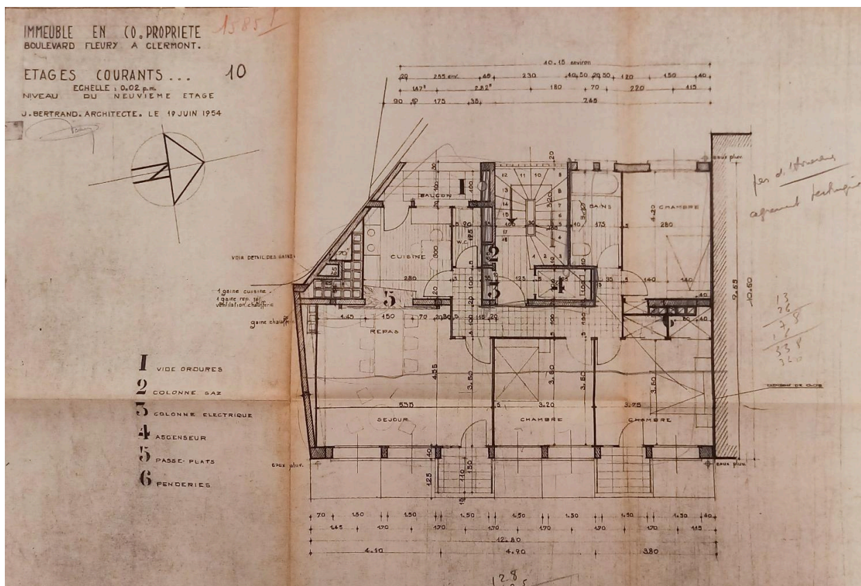
Plan d'étage courant (1954)
