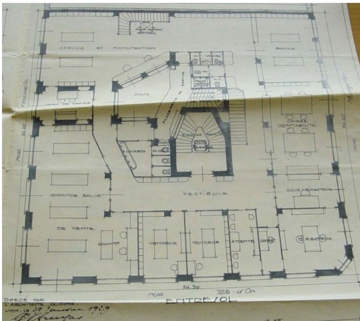
Plan de l'entresol
