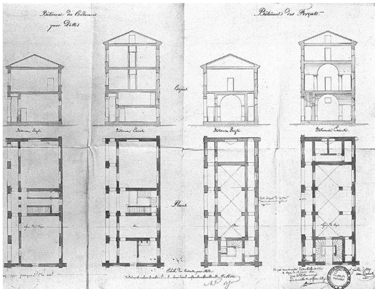
Plans et coupes du bâtiment des condamnés pour dettes et du bâtiment des forçats, par l'architecte Dumont, 16 juillet 1829. 49,5 x 65 AD, Rhône. 1 Y 299
