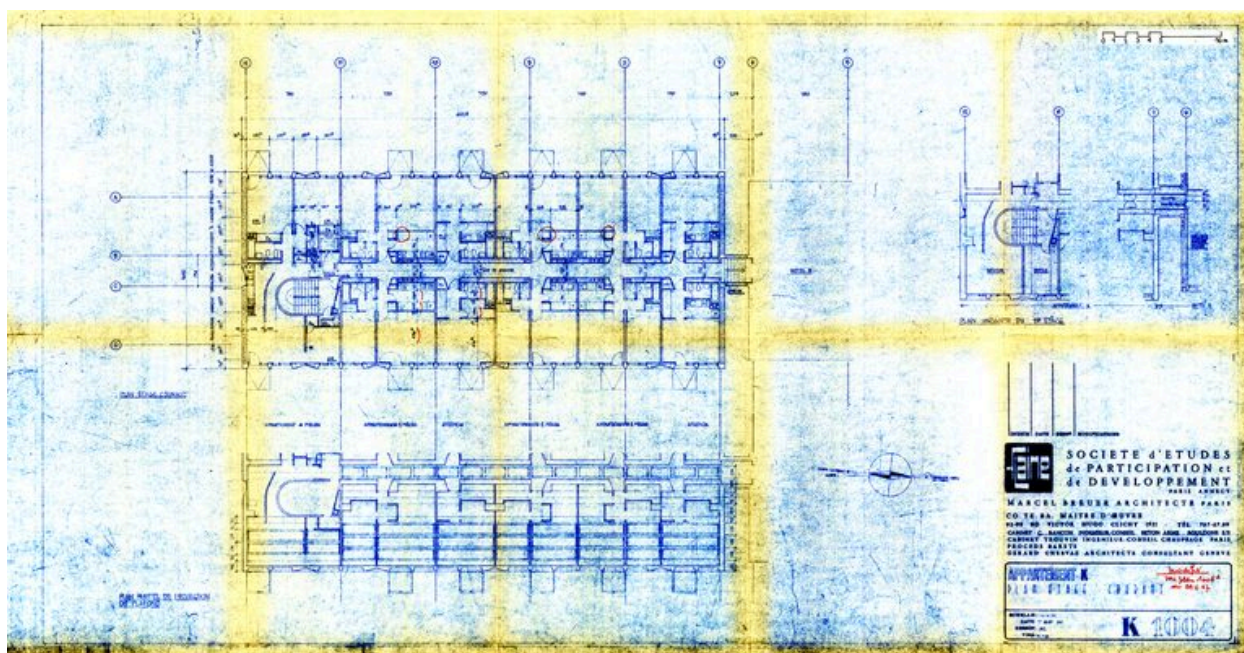
Appartement K. Plan d'un étage courant. Marcel Breuer architecte, 10 septembre 1966 (AC Arâches-la-Frasse)
