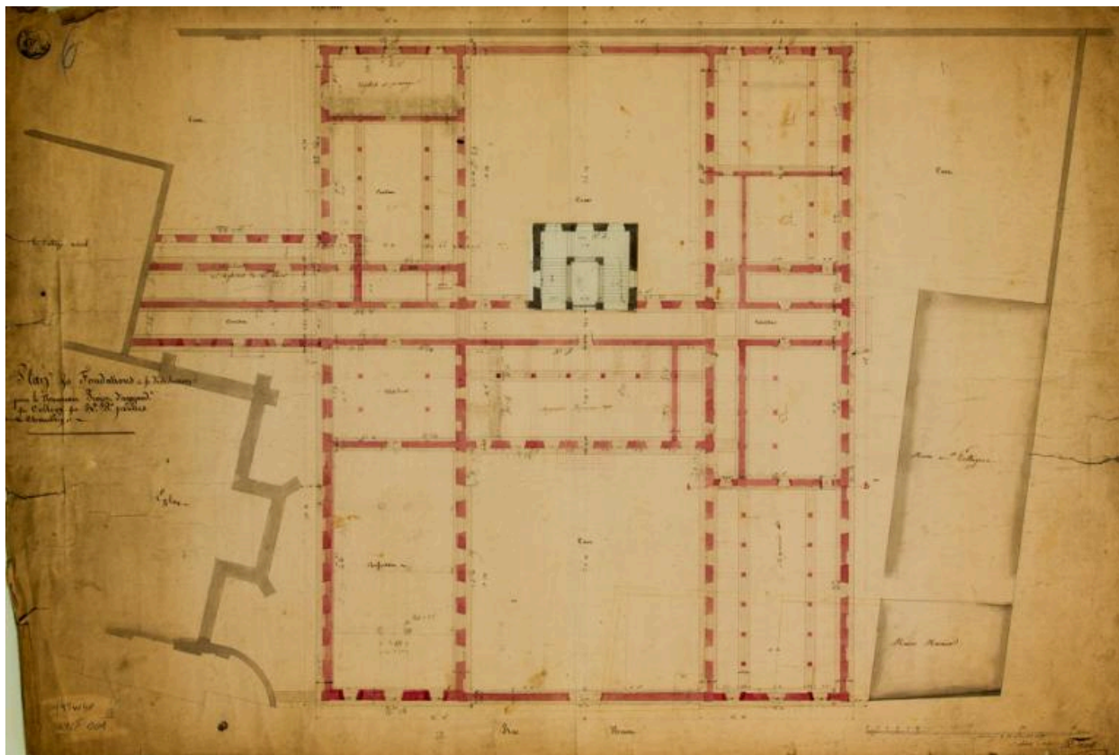
Plan des fondations et de distribution. 1827.
