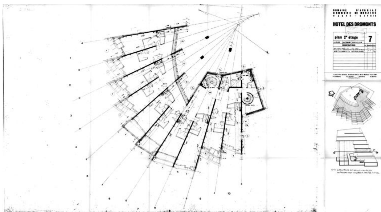
Projet Jacques Labro. Plan du 2e étage / J. Labro, 14 juin 1965 (AC Morzine)
