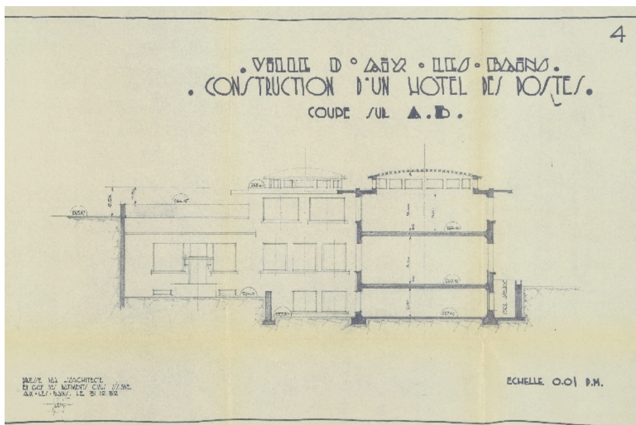
Coupe AB
