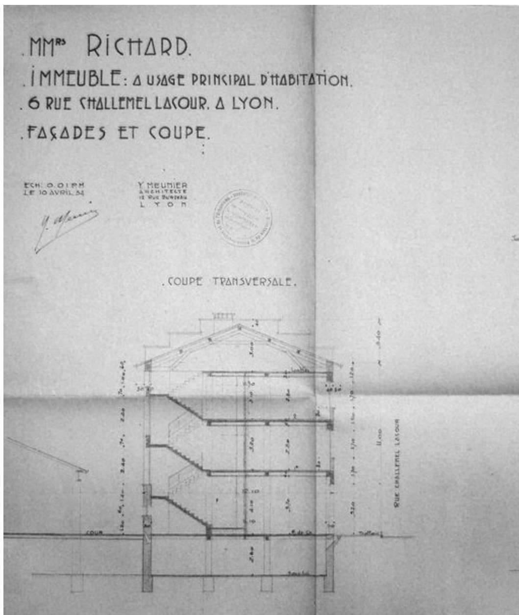
Coupe transversale, Immeuble à usage principal d'habitation, 6 rue Challemel Lacour, 10 avril 1954 par Yvon Meunier architecte, échelle 1/100. (Arch. mun. Lyon)
