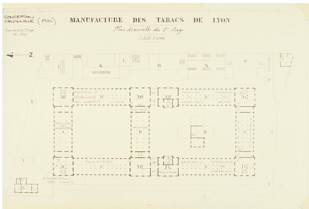
La Manufacture des Tabacs de Lyon. Plan d'ensemble du 1er étage. Conception originale (1910)
