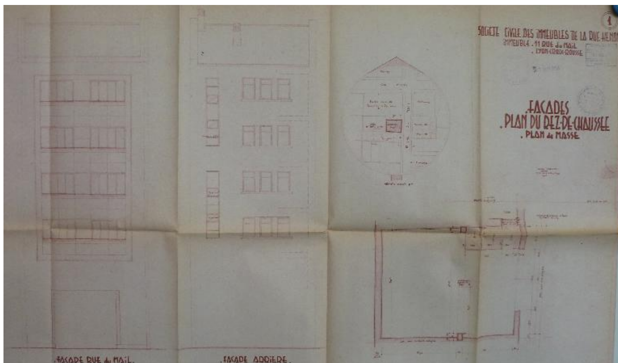
Elévations et plan du rez-de-chaussée (Arch. Mun. Lyon, 345 W 080 : Permis de construire, 1925)
