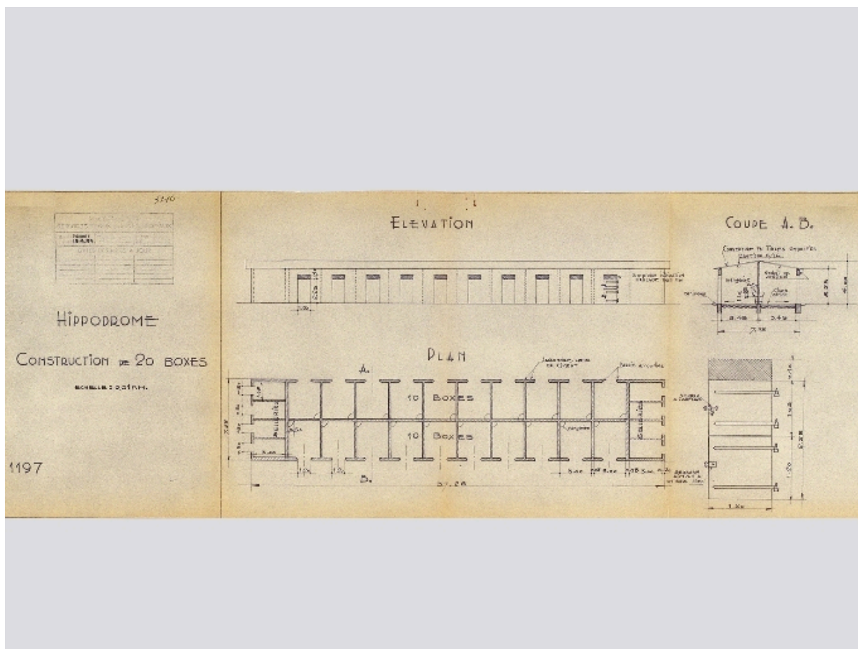
Plan, coupe et élévation d'une écurie, 1959
