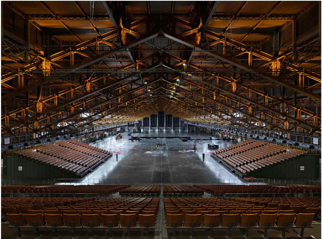
Vue d'ensemble du grand système de charpente métallique
