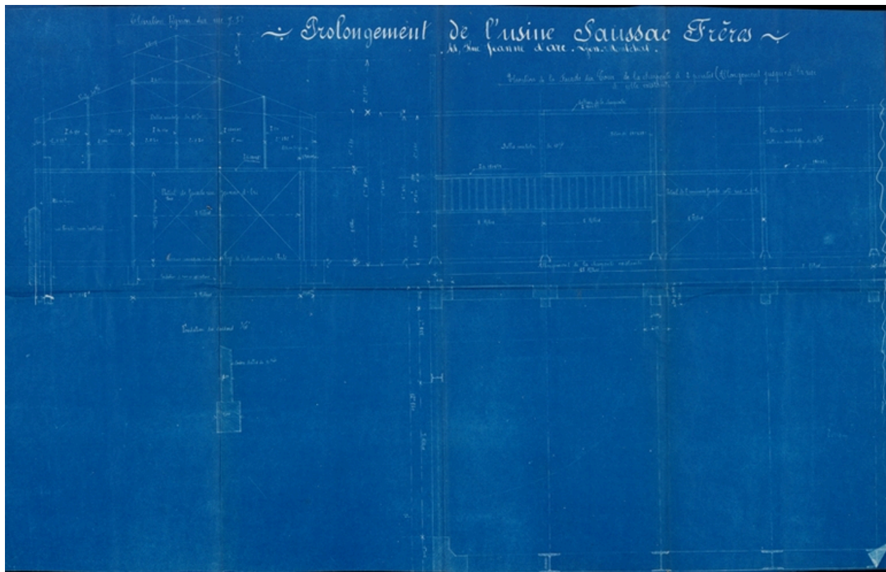
Plan et coupe de l'agrandissement de l'usine de messieurs Saussac Frères, 1925. AC Lyon : 344 WP 178 PCA n°0570
