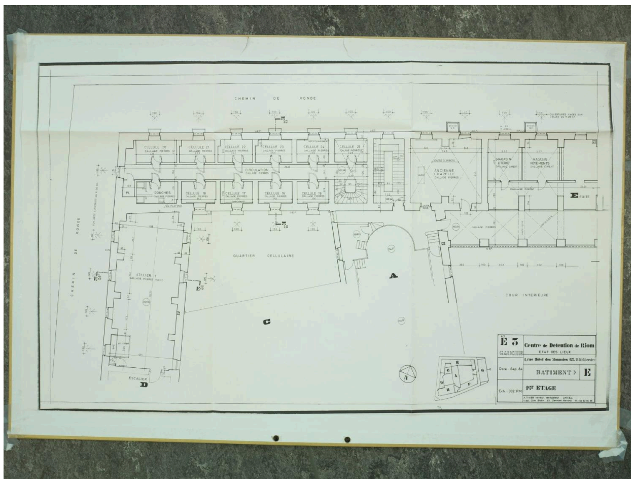
Bâtiment E, plan, 1er étage, gauche, éch. 002 p.m. État des lieux, septembre 1984.
