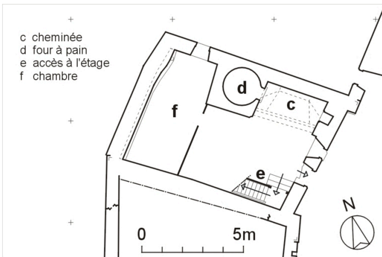
Logis ancien. Plan du rez-de-chaussée. Relevé manuel expédié.
