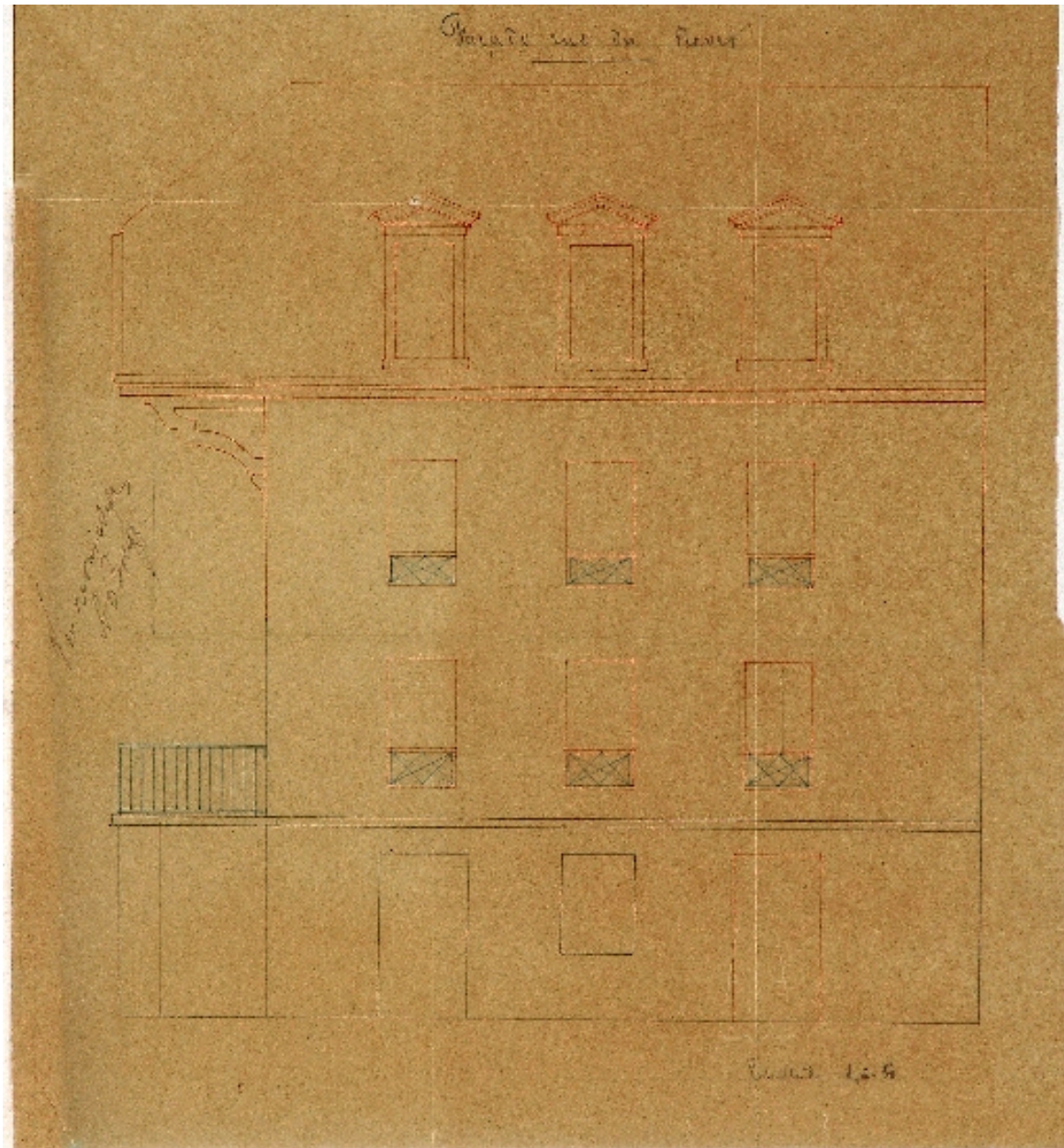
Élévation de la façade principale
