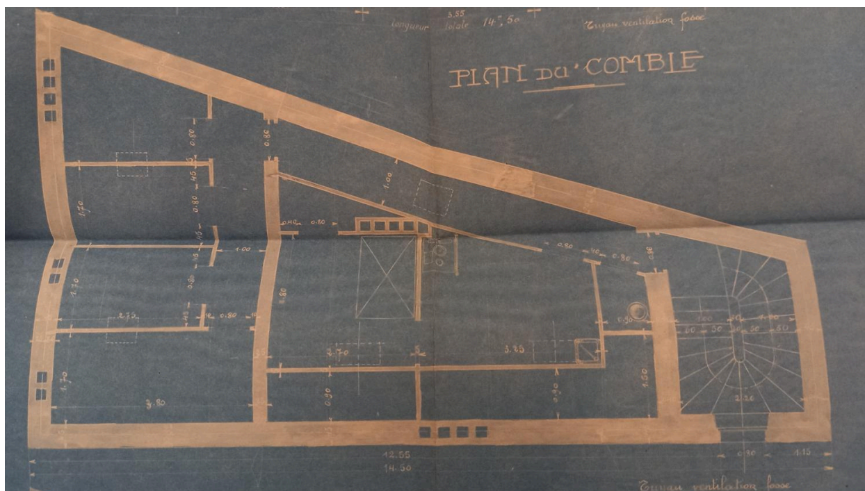
Plan des combles, 24 avenue d'Italie
