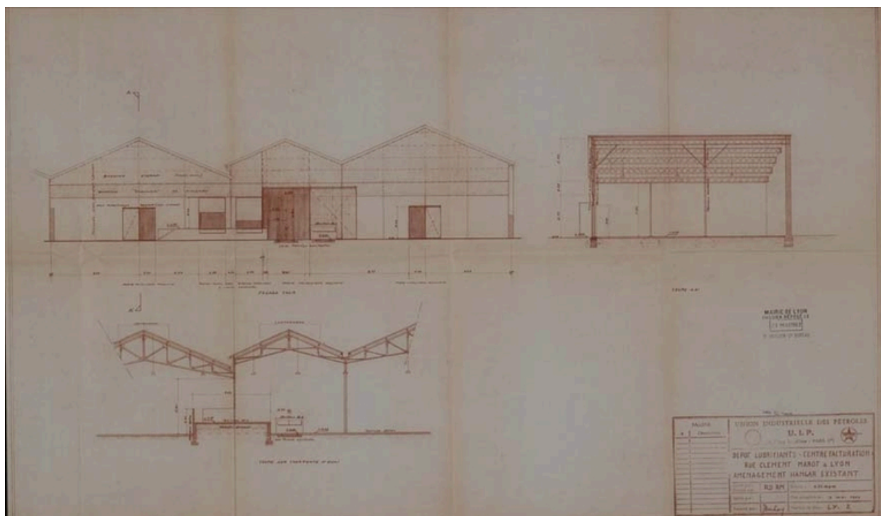
Plan d'aménagement d'un hangar (coupes et façades) 1934
