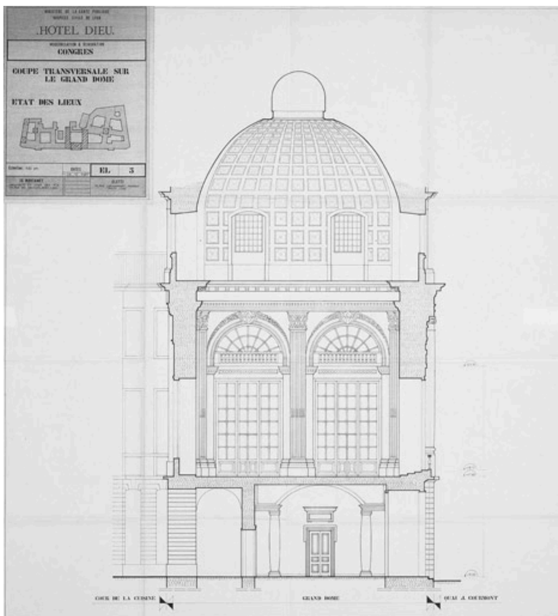
Modernisation et rénovation. Congrès. Coupe transversale sur le grand dôme, état des lieux, Mortamet/ SLETTI, 26/12/1977
