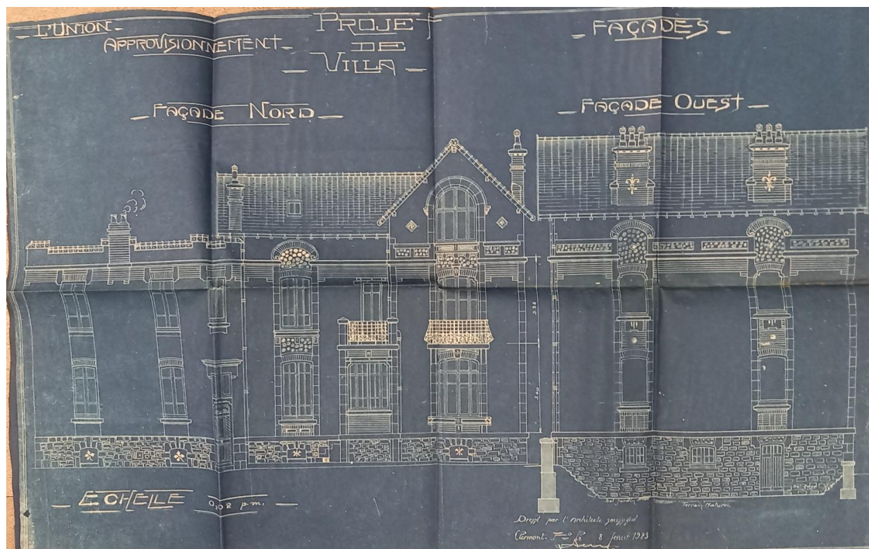
Façade sur le boulevard Cote-Blatin et élévation latérale
