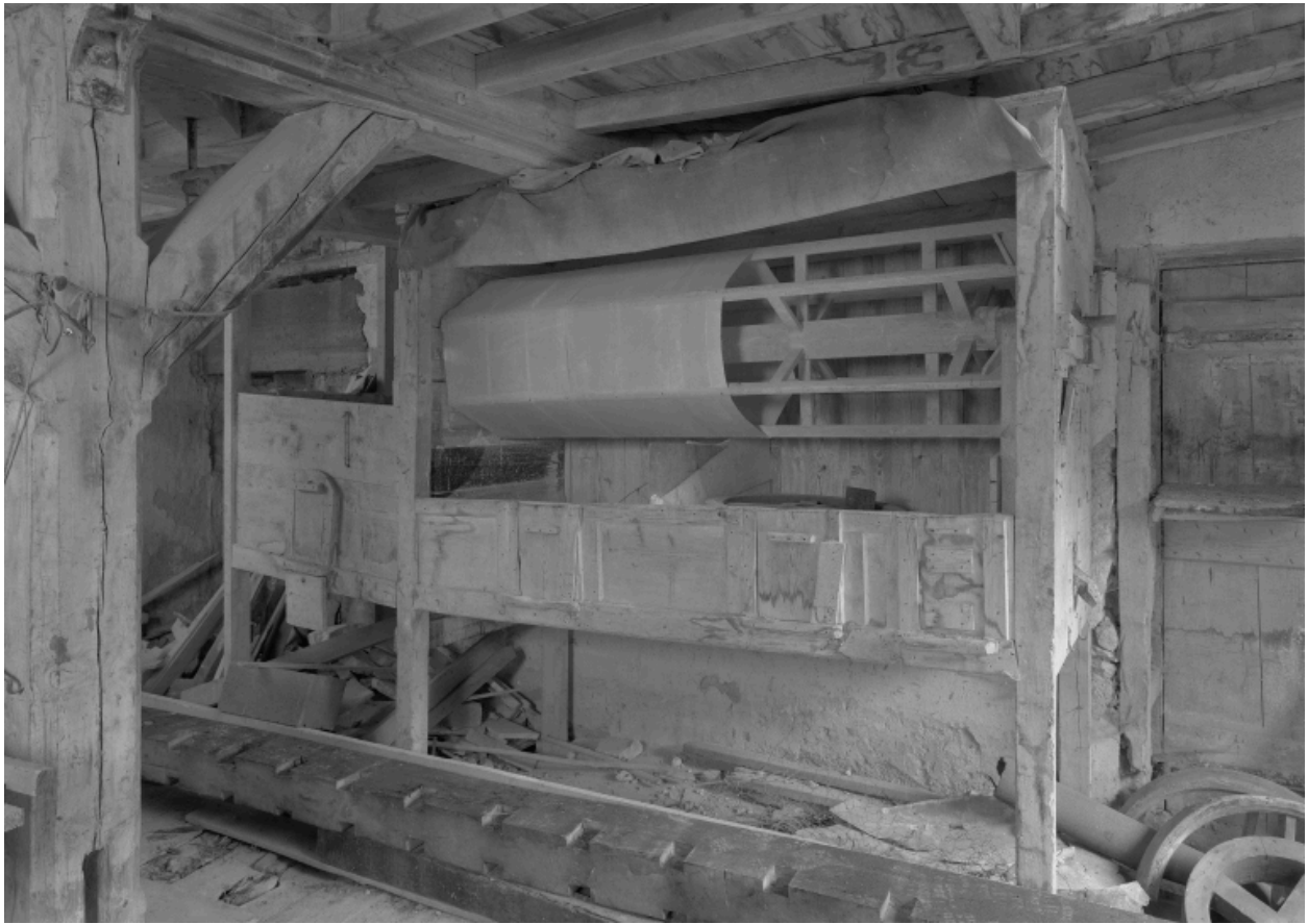
Intérieur du moulin, rez-de-chaussée, tamis.
