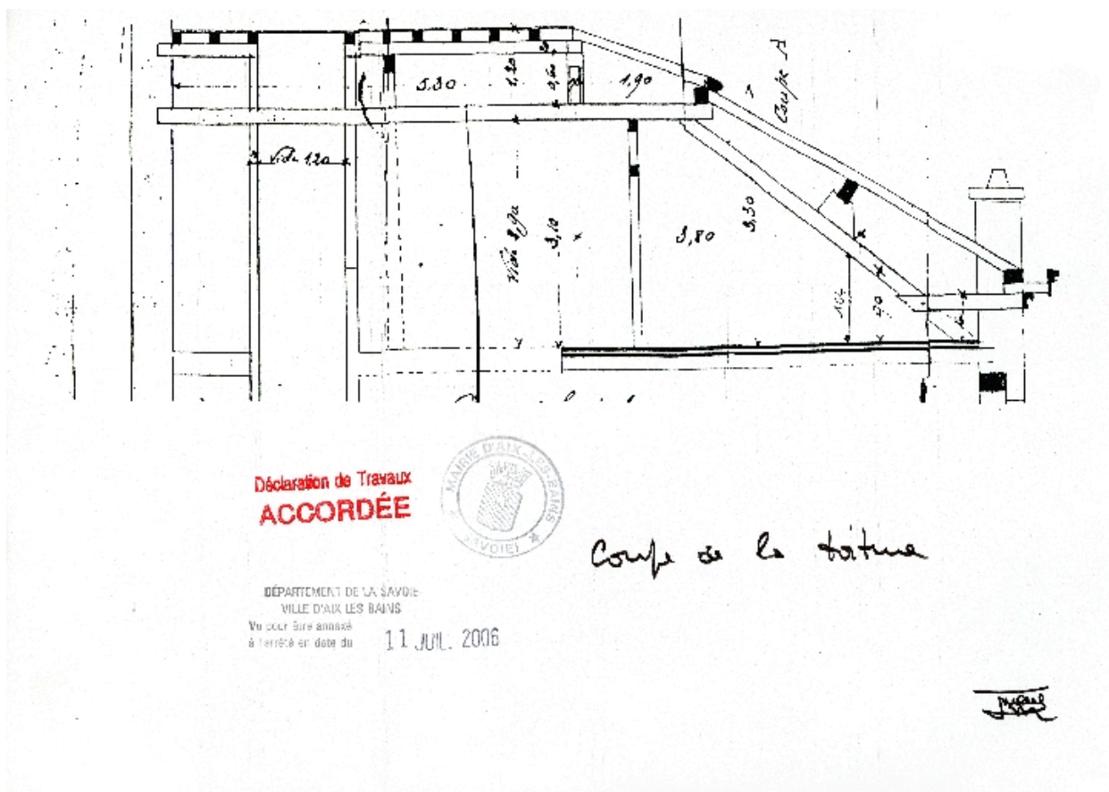
Coupe de la toiture, 2006
