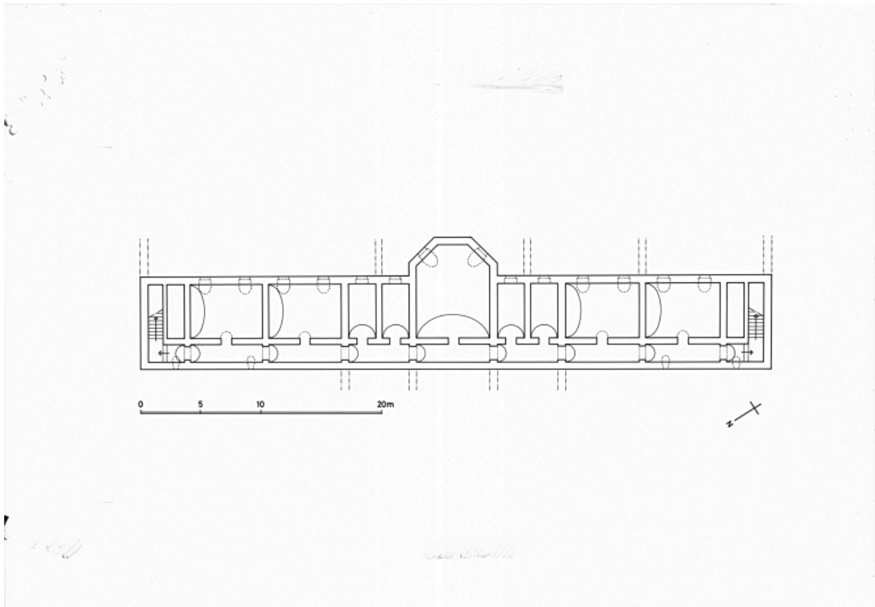
Plan du sous-sol, d'après Constancin, 1983. Dessin Inv. P. Cherblanc, 1996
